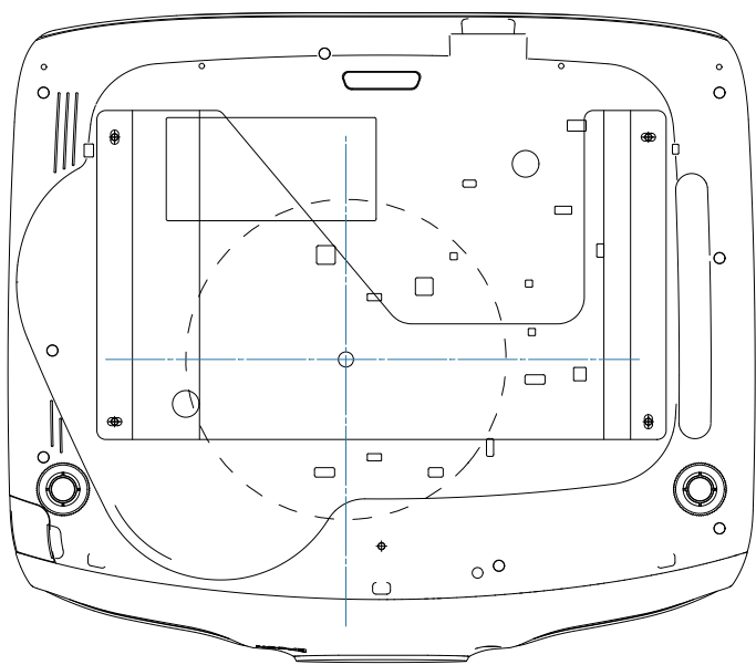
EH-TW6000/TW6000W天吊金具(ELPMB20)装着图
