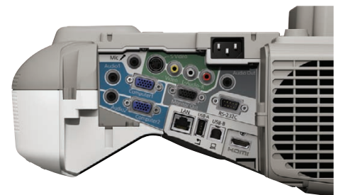
Anschlussfeld des Epson EB-475Wi
