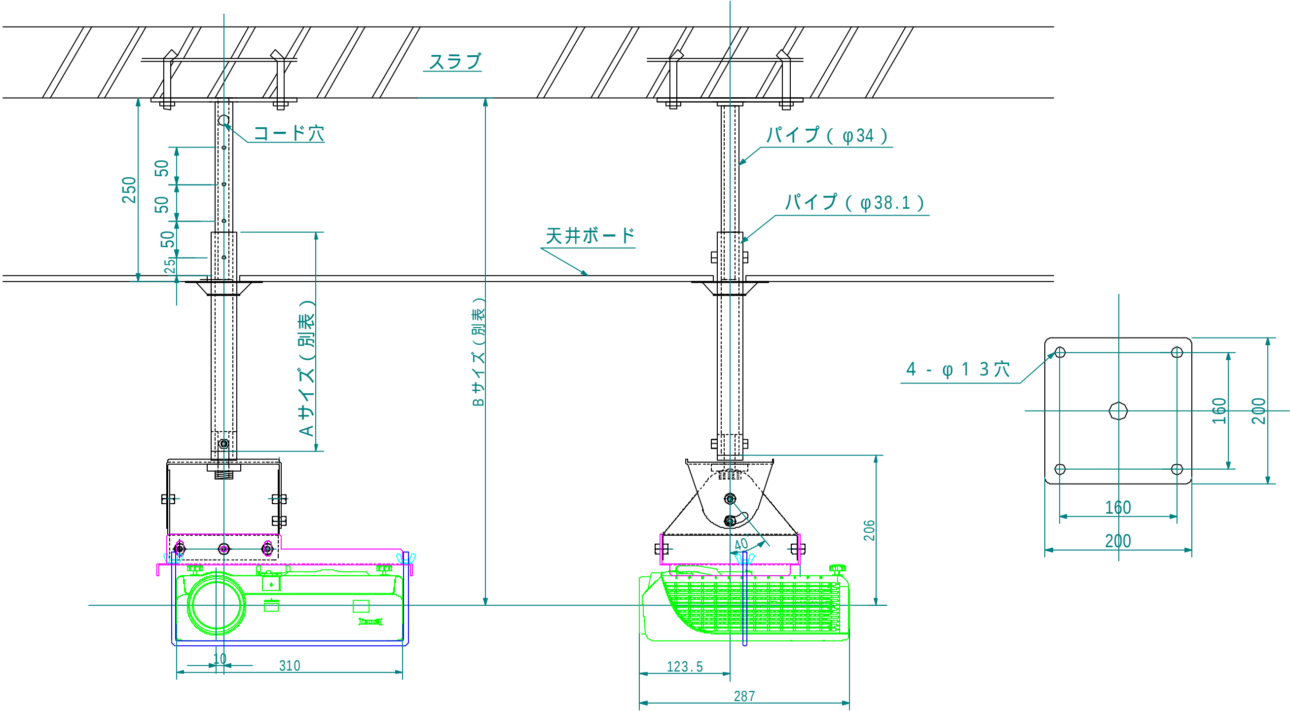
(パイプ)
